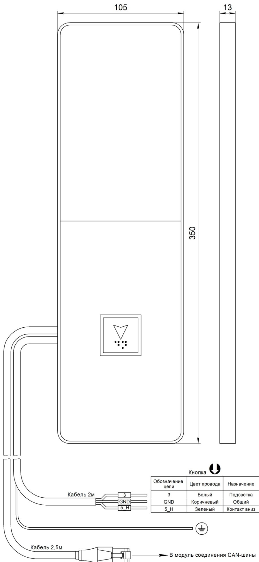
Рис.1 Внешний вид, габаритные и установочные размеры Вызывного поста МАЛАХИТ (жгут RJ45) НШЕК.468381.086
